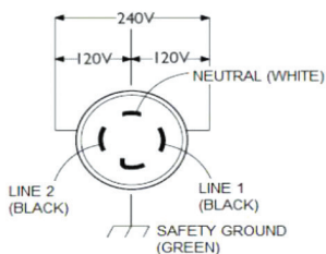
Extension 240V à fournir par le client
